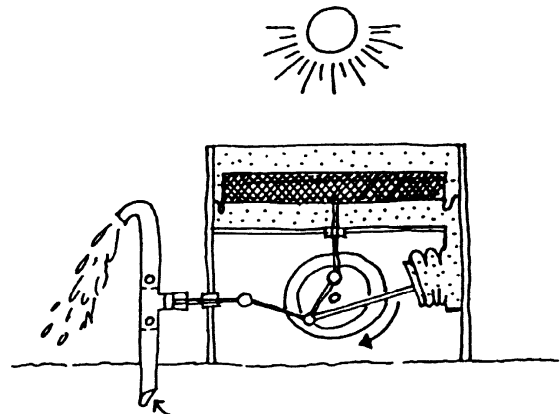
Einfacher Solar-Stirlingmotor als Wasserpumpe
