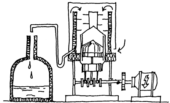
Stirling-Luftverflüssiger
