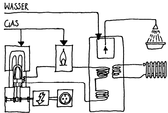
Stirling-BHKW für Mehrfamilienhäuser (Komplett-Anlage)
