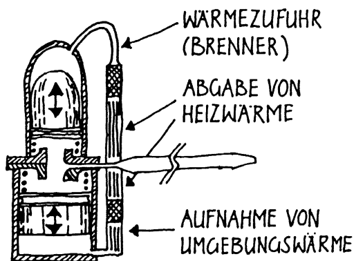
Vuilleumiermaschine
