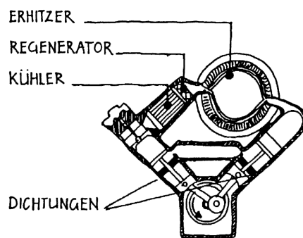
Anspruchsvolle Bauteile im Stirlingmotor
