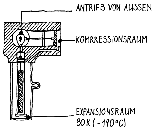
Kleines Kühlaggregat für Infrarotsensoren
